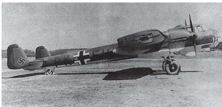
Бомбардировщик Do 215 (Германия)
